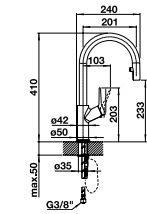
Kaltstart Auslauf 190° schwenkbar mit umstellbarer Schlauchbrause
