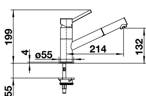
Kaltstart Auslauf 120° schwenkbar mit Schlauchauszug
