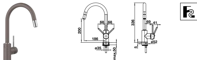
Auslauf 360° schwenkbar mit Schlauchauszug
