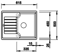
Ausschnitt: 595 x 480 mm Beckentiefe: 190 mm Außenmaß: 615 x 500 mm Mindesteinbauhöhe: 333 mm
