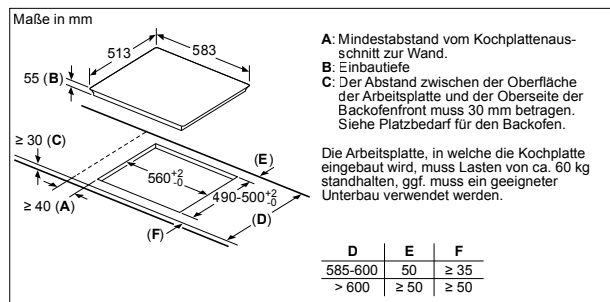
NXX645CB5E | NVS645CB6E – umlaufender Edelstahl-Rahmen
