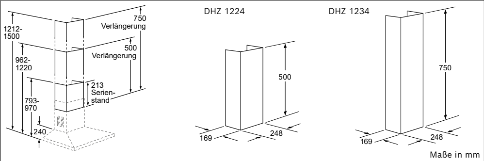
Sonderkanäle für Wandessen DHZ1224 | 1234
