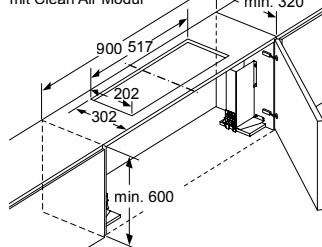
Montage Flachschirmhaube mit Clean Air Modul
