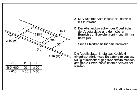
PXE845HC1E – umlaufender Rahmen
