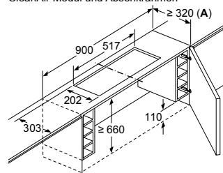
Montage Flachschirmhaube mit CleanAir Modul und Absenkrahmen
