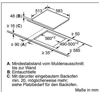
PKN645BA2E – umlaufender Rahmen
