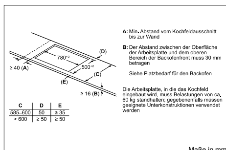
PXV845HC1E – umlaufender Rahmen
