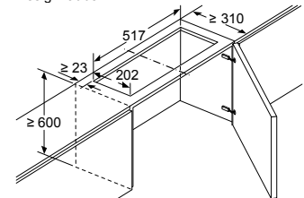
Montage Clean Air Modul mit integrierter Designhaube
