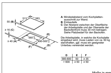
PXX645HC1E – umlaufender Rahmen
