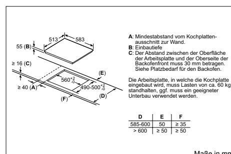
PIE645BB5E – umlaufender Rahmen
