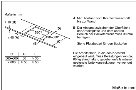
PVS645HB1E – umlaufender Rahmen
