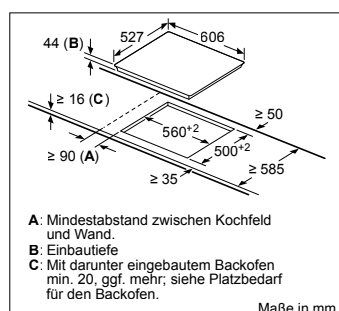
PKN675DP1D – Comfort Profil
