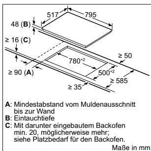
PKH845BB1D – umlaufender Rahmen
