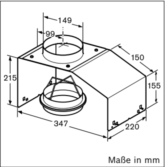
Montagehilfe DHZ7402
