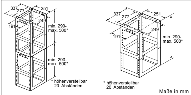
Montageturmverlängerungen DHZ1253 | 1251
