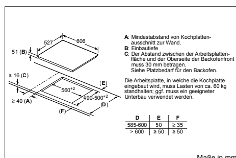
PXX675DC1E – Comfort Profil
