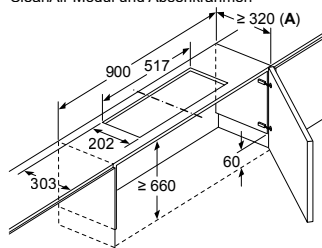
Montage Flachschirmhaube mit CleanAir Modul und Absenkrahmen
