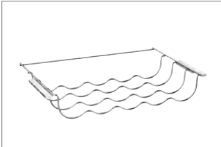
KSZ10020 Verchromte Flaschenablage für Einbaugeräte, passend für: KIR21, KIL22, KIR31, KIL32, KIR41, KIL42, KIF4, KIF5, KIL72, KIR81, KIL82 UHP: 81,- €*
