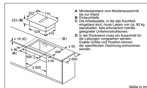
PVQ711H26E - Rahmenlos aufliegend (nicht flächenbündig einbaubar)
