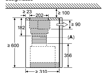
Montage Clean Air Modul mit integrierter Designhaube
