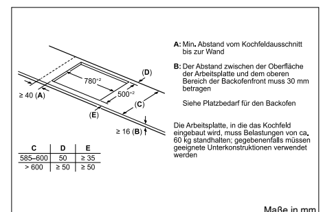
PIV845HB1E – umlaufender Rahmen
