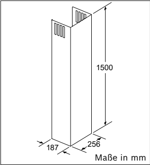
Sonderkanäle für Wandessen DWZ0AX5L0
