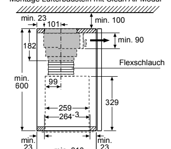
Montage Lüfterbaustein mit Clean Air Modul
