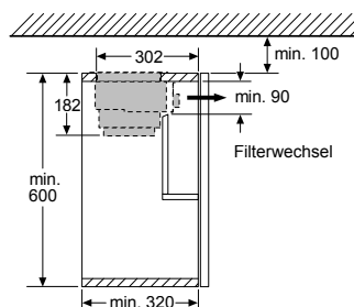
Montage Flachschirmhaube mit Clean Air Modul
