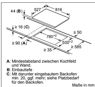
PKM875DP1D – Comfort Profil
