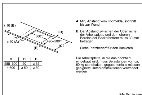
PIX645HC1E – umlaufender Rahmen
