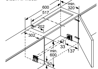
Montage Flachschirmhaube mit Clean Air Modul
