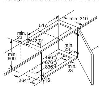
Montage Lüfterbaustein mit Clean Air Modul
