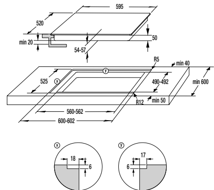
ECD 643 BSC Flächenbündig
