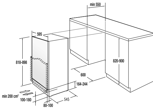
RBIU 609 FA1 / RIU 609 FA1
