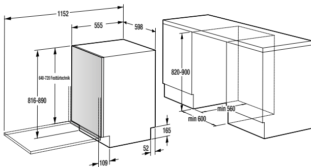
GV 693 C60UVAD / GV 642 D61 / GV 663 D60
