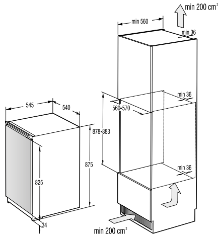
RBI 4092 E1 / RI 4092 E1 / FI 4091 E1
