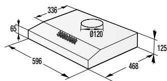
WHU 629 ES/S / WHU 629 EW/S
