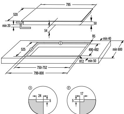
IS 846 BG Flächenbündig
