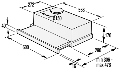
TH 64 E3BG / TH 60 E3X
