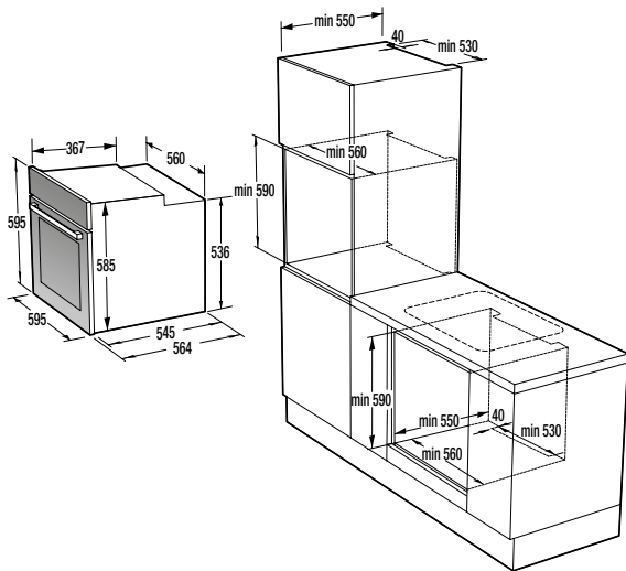
BPSA... / BSA ... / BPS... / BPSX... / BOS... / BOSX... / BO...
