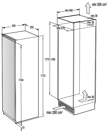
RBI 5182 A1 / RI 518 EA1 / FNI 518 EA1
