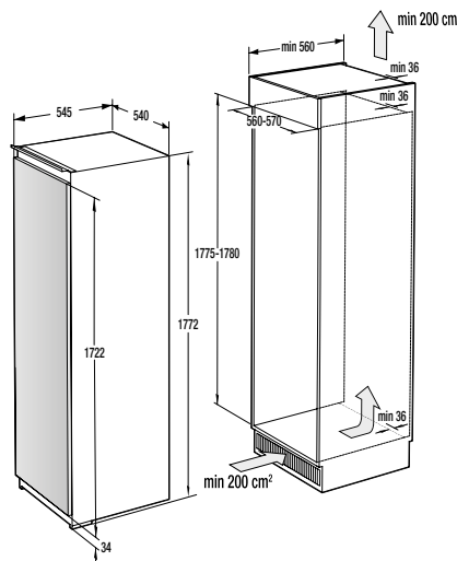
RBI 4182 E1 / RI 4182 E1
