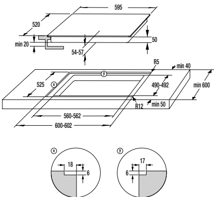
ECS 646 BCSC / ECT 643 BSC Flächenbündig
