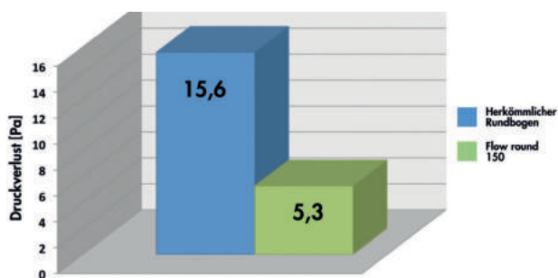
Geringerer Druckverlust bei COMPAIR® flow round 150
