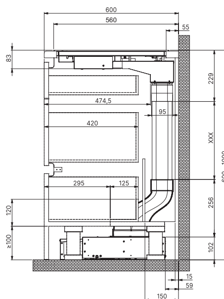
Einbau Umluft mit Kohlefilter im Sockel
