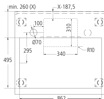
Ausschnittsmaße APL- und Unterschrankboden
