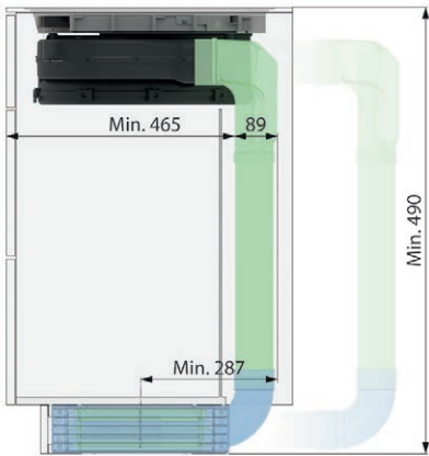
Für seitliches Ausblasen der geführten Umluft mit liegendem Filter.
