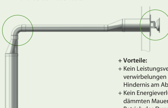
berbel Flachrohr-System und berbel Mauerkasten
