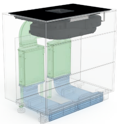
U2 mit Luftaustrittsgitter vorne, Umluftfilter stehend
