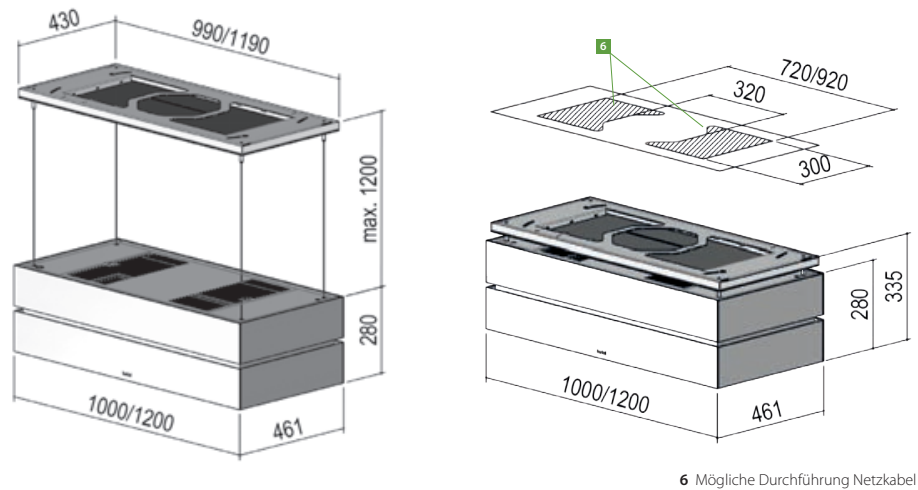
6 Mögliche Durchführung Netzkabel
