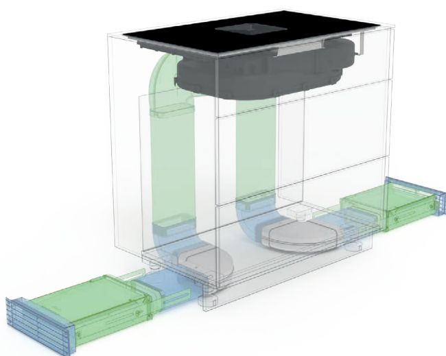
U5 mit Luftaustrittsgitter seitlich, Umluftfilter liegend
