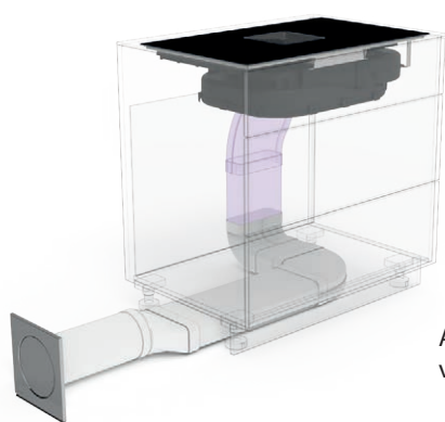
Abluftführung in der Tiefe variabel positionierbar.
