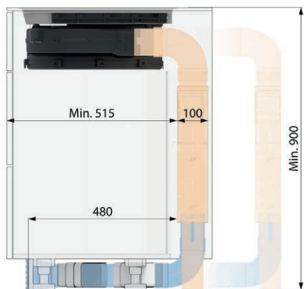
Kürzester Weg der Umluftführung aus dem Möbel mit stehendem permalyt®-Filter.
