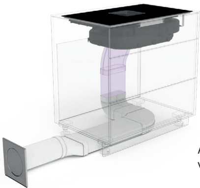
Abluftführung in der Tiefe variabel positionierbar.
