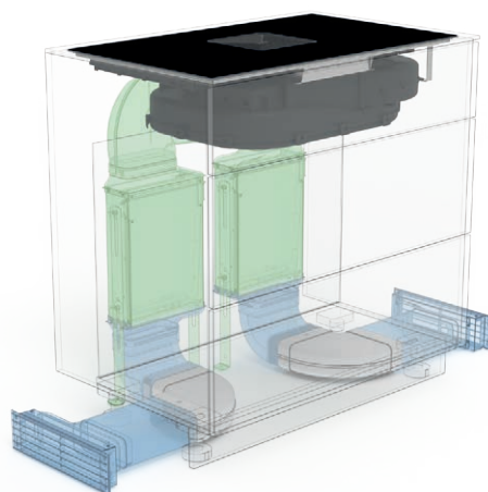
U3 mit Luftaustrittsgitter seitlich, Umluftfilter stehend
