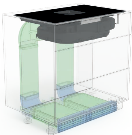
U4 mit Luftaustrittsgitter vorne, Umluftfilter liegend
