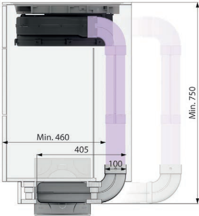
Mit kompakter Einbautiefe durch Einsatz des Doppelbogens
