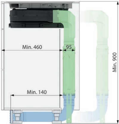
Kürzester Weg der Umluftführung aus dem Möbel mit stehendem Filter.
