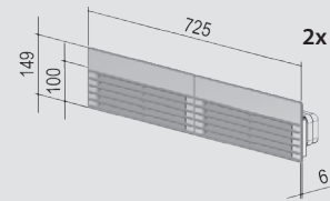
(Abbildung zeigt Luftführung nach vorne)
