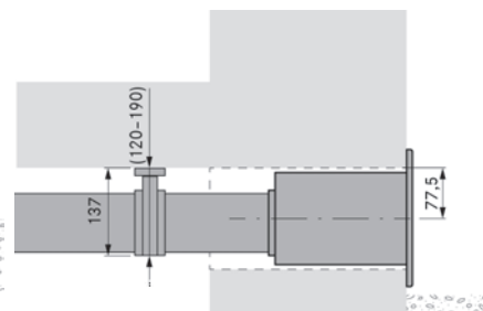
Kanalführung an Kellerdecke
