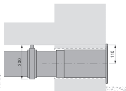
Kanalführung an Kellerdecke
