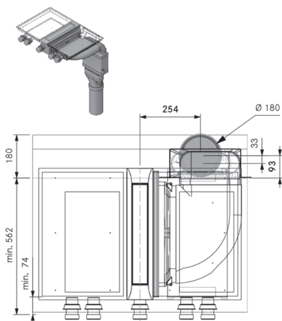
PKA3 mit Flachschalldämpfer USDF und Übergangsstück gerade EFRG (Insel)
