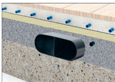
Flachkanal in der Ausgleichsschicht (nach DIN 18560-2)
